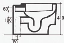
VASO / TOILET
